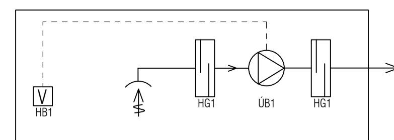
KERFI 1-3 - ÚTSÖGSKERFI FYRIR GEYMSLUGANGA, HJÚLA-VAGNAGEYMSLU OG TÆKNIRYMI Í KJALLARA.
