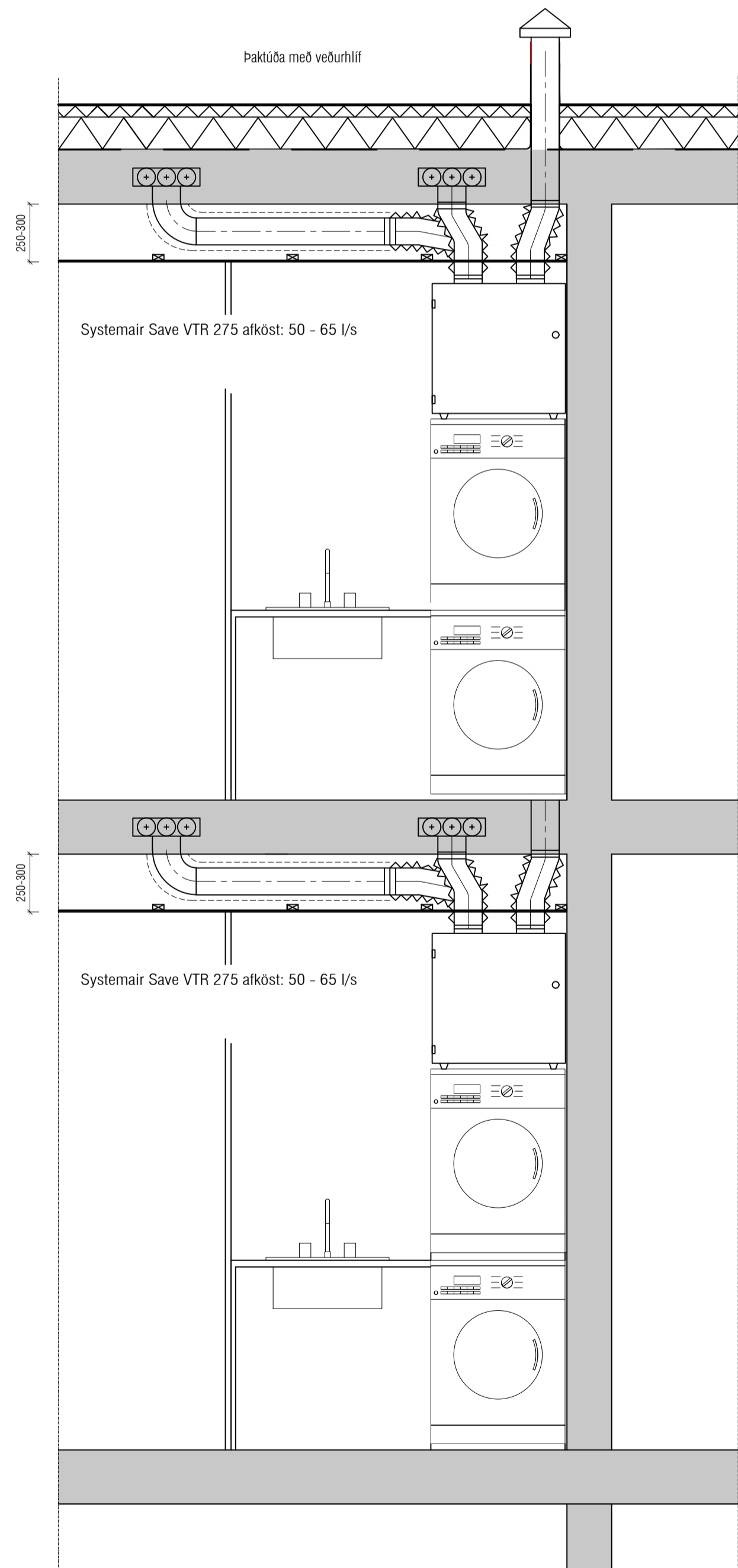
DÆMIGERT SNÍÐ AF BAD I/ BVH 1:20
